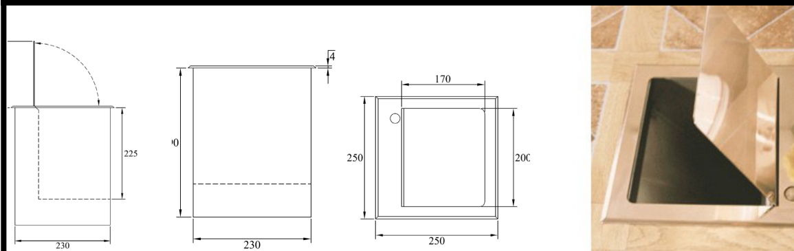
Garbadge Chute/ Afvalluikje H45.03
